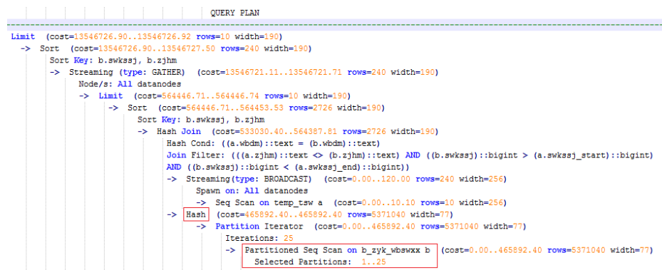
图 13-7 应用 unlogged table 案例（二）
