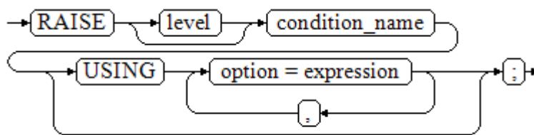
图 9-35 raise_condition::=
